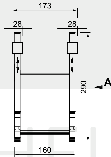
Ansicht B
