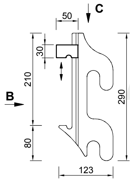
Ansicht A
