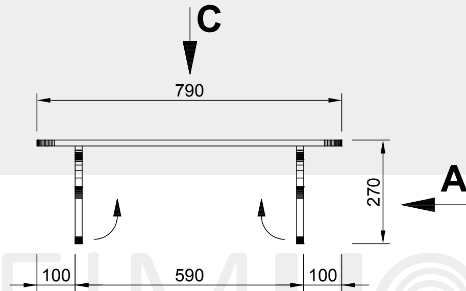
Ansicht B
